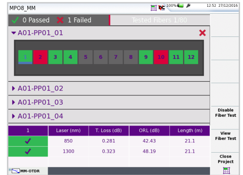
图 3. OTDR 光开关界面
