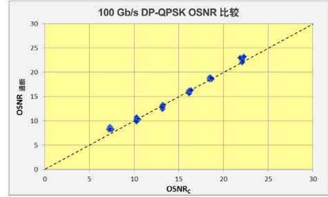
图 6: 100 Gb/s OSNR 比较
