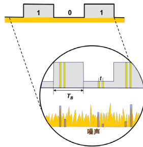
图 3：相关性测量
