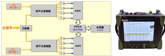
图 5: OSA-710 方框图
