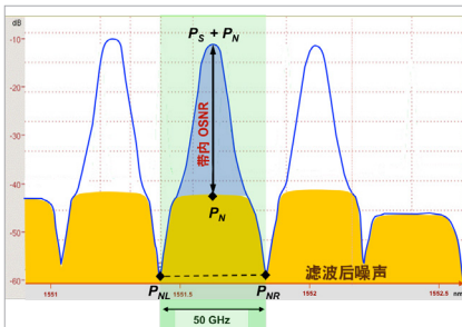
图 2: ROADM 系统中滤波噪声的影响
