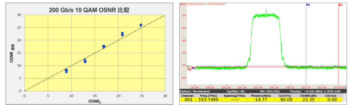
图 7: 尼奎斯特信号和 OSNR 结果
