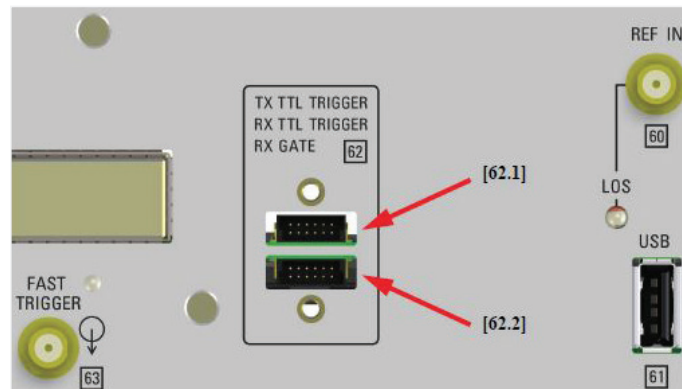
图 4. ONT CFP2 模块输出针脚
