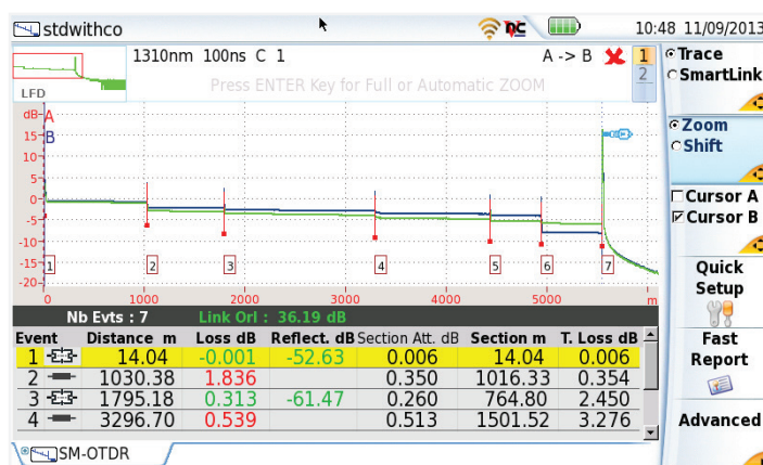
OTDR 迹线视图
