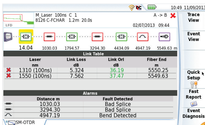
基于图标的 OTDR 结果视图
