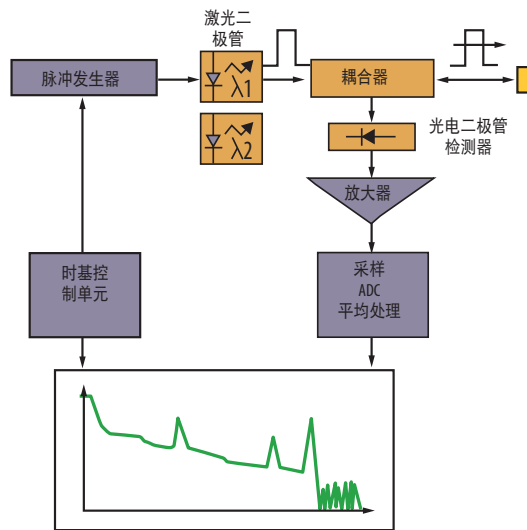
OTDR 原理框图
