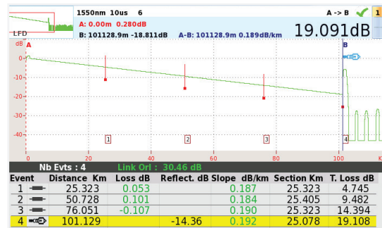
光纤链路的图示，也称为 OTDR 迹线
