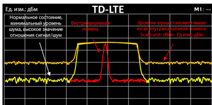
Рисунок 1. Сигнал LTE-TDD с помехами
