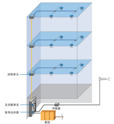
DAS 架构示例
