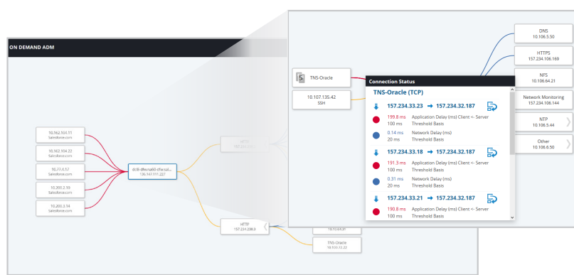
Diagramme mit automatischer Anzeige der Abhängigkeiten zwischen Anwendungen (ADM) und integriertem Endnutzer-Scoring (EUE)
