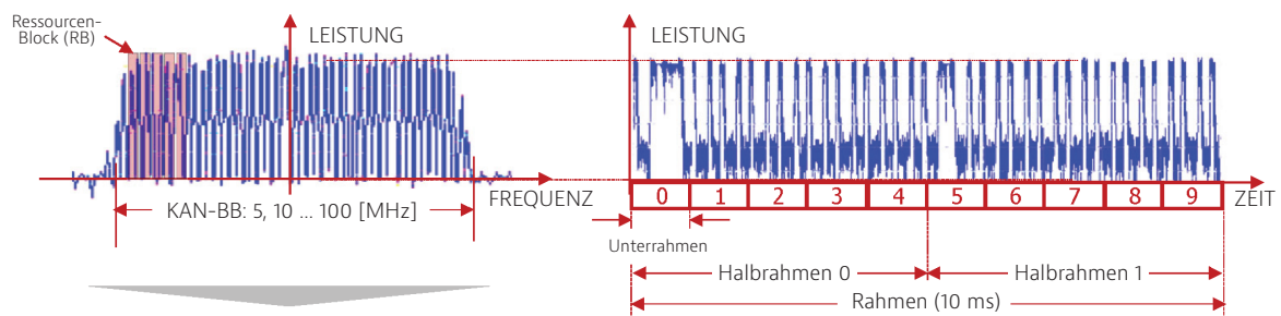
Signalkanal und Rahmenstruktur von 3GPP 5G NR
