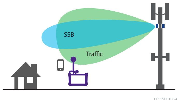
Codeselektive EMVU-Messung im 5G-Netz an Traffic-Beams bei einer Highspeed-Datenübertragung
