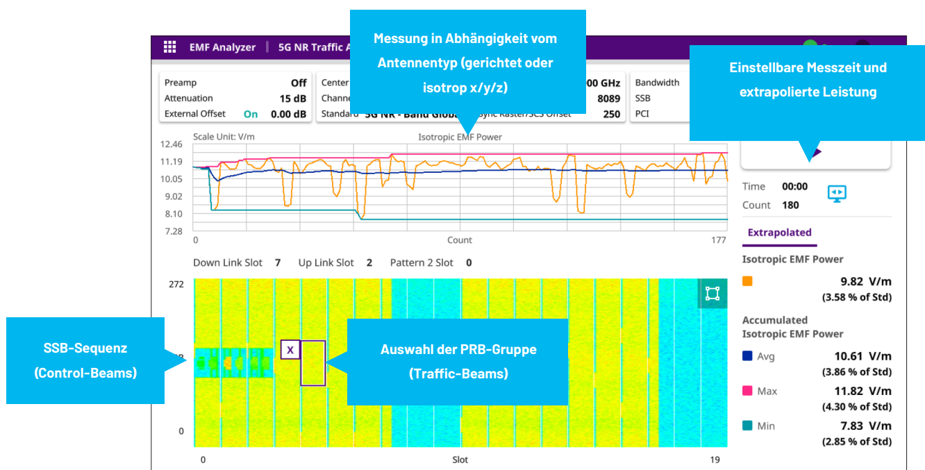
5G EMVU-Verkehrsanalyse mit dem OneAdvisor 800 Wireless im codeselektiven Modus
