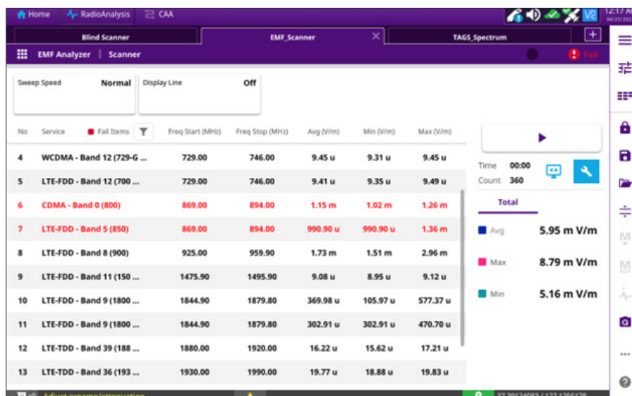
EMVU-Scanner-Messung mit dem OneAdvisor 800 Wireless im frequenzselektiven Modus
