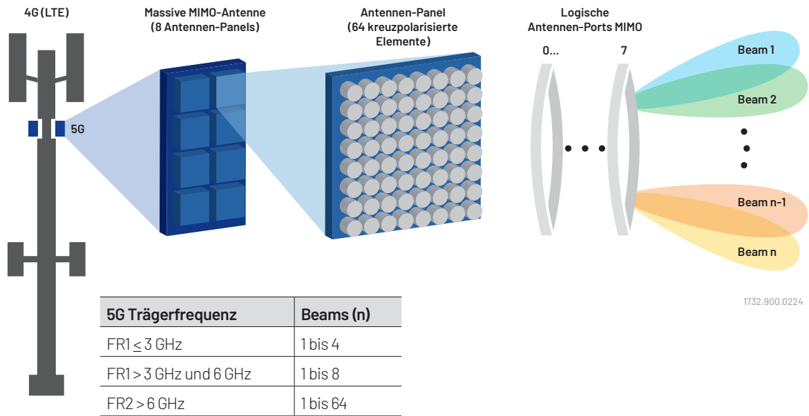
5G Massive MIMO und Beamforming
