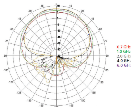
H-plane
