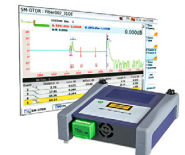
● Módulos da Série 4100 OTDR padrão, OTDR FiberComplete CWDM/DWDM e chave óptica MPO OSA/OCC
