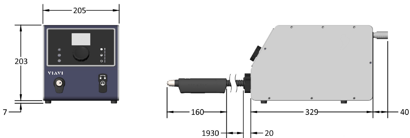
Figura 5: Dimensiones del sistema CleanBlastPRO
