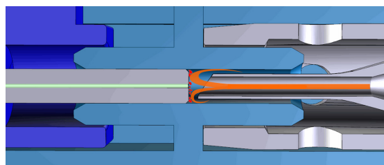
Figura 1b: Procedimiento de limpieza sin contacto optimizado
