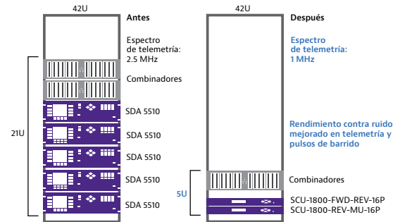
El SCU-1800 ahorra espacio en rack y disminuye el uso de redes combinatoras con los 16 puertos disponibles para el barrido de reversa
