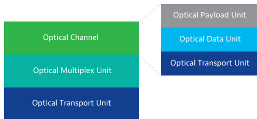
Figure 19: OCh substructure and basic OTN structure
