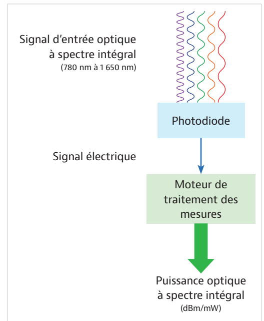
Figure 1 : Schéma de photomètre optique large bande
