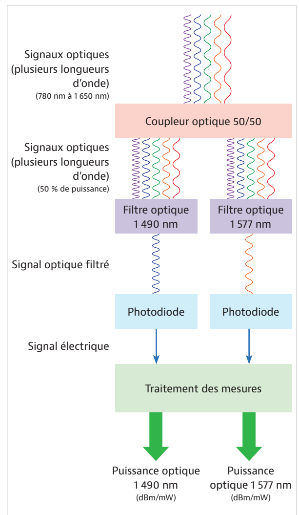
Figure 2 : Schéma d'un photomètre optique sélectif
