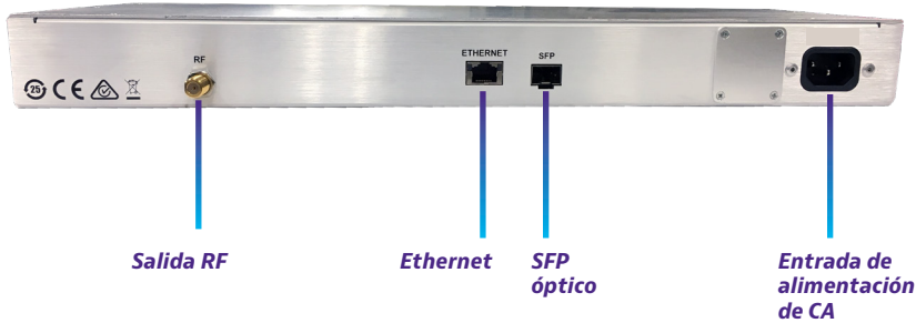
Modelo de alimentación de CA
