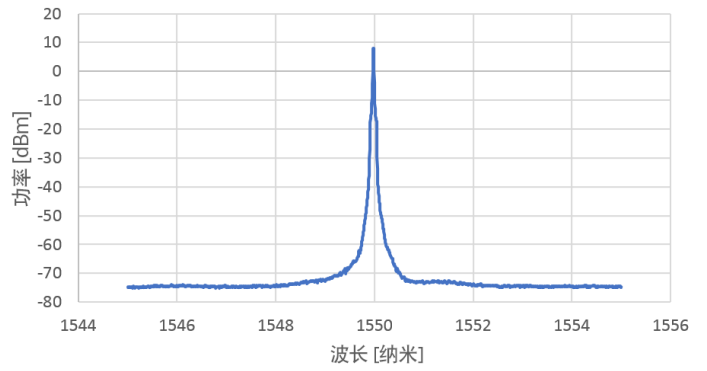
图 2: mTLS-C1 噪声电平
