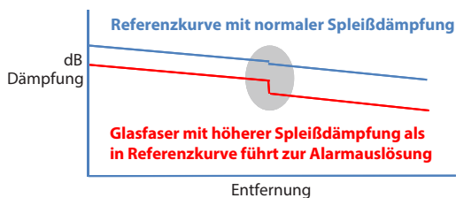
Anzeige eines angezapften Spleißes in der OTDR-Kurve
