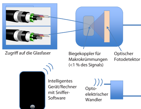
Prinzipielle Vorgehensweise beim Anzapfen einer Glasfaser
