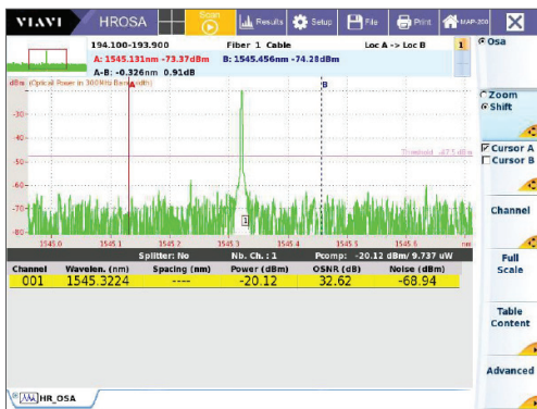
带有以表格形式呈现的波长、功率和低分辨率图表的波长计 GUI
